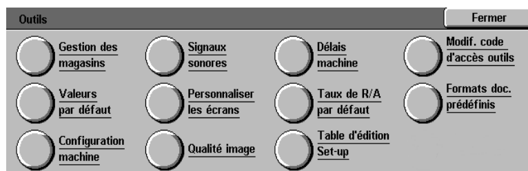
Figure 5 : menu-écran Outils
