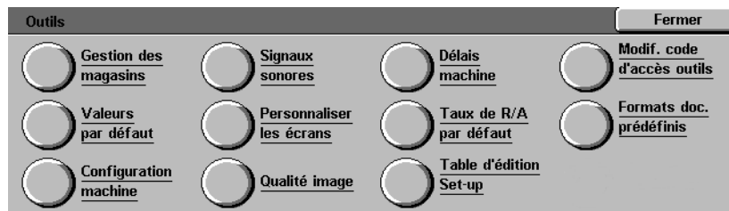
Figure 1 : menu-écran Outils
