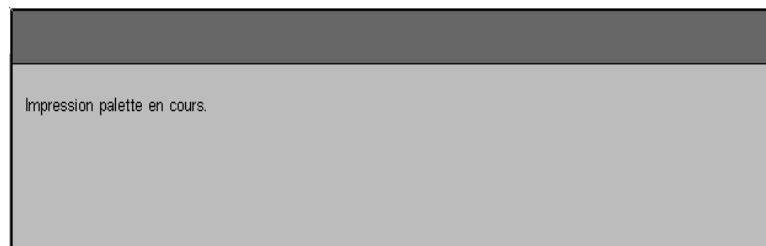
Figure 11 : message d'impression
