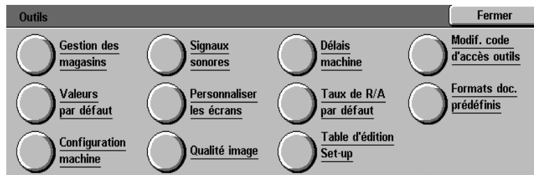
Figure 12 : menu-écran Outils
