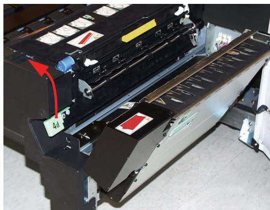
Griff 4d nach oben drücken
