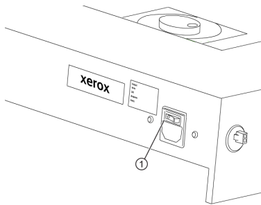
1. Betriebsschalter
