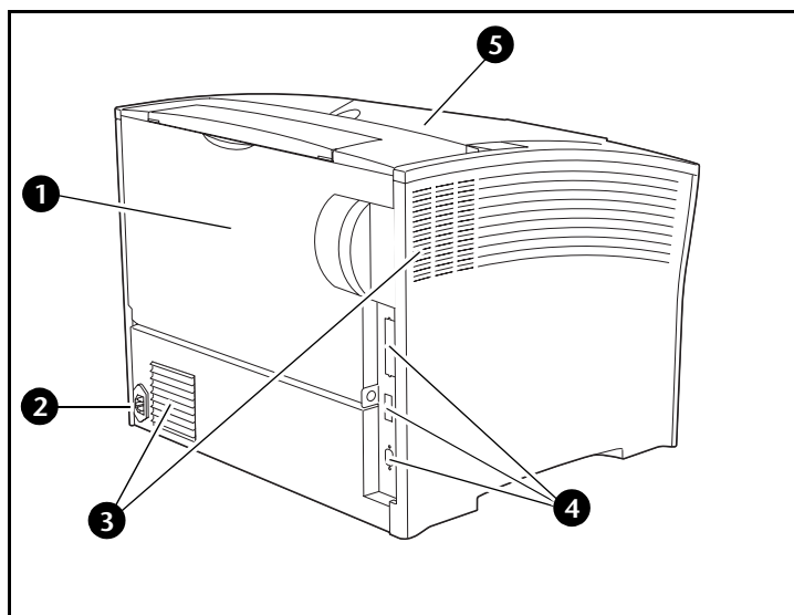
Abbildung 1.2 Druckerkomponenten, Rückansicht
