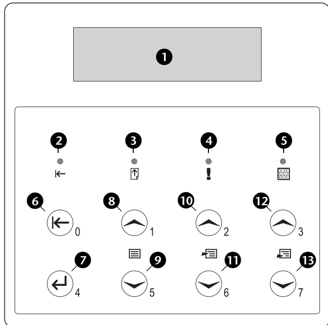
Abbildung 3.1 Bedienfeld 1
