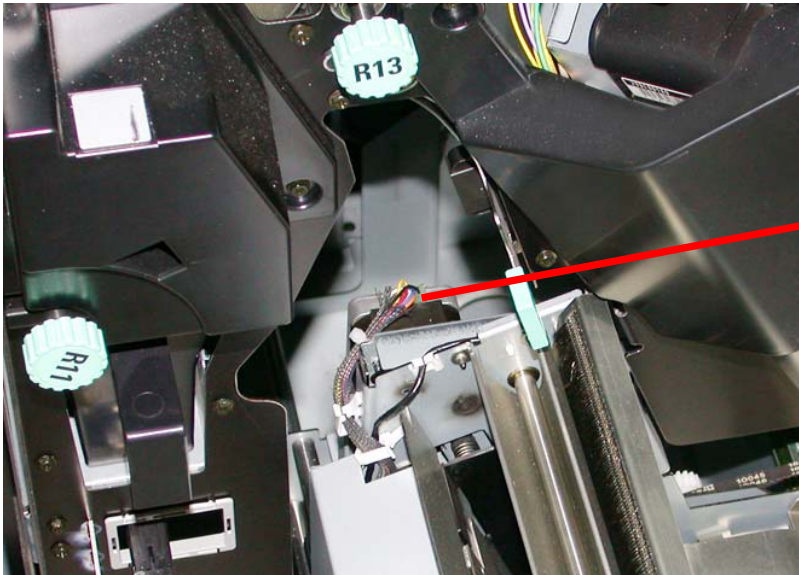
Abbildung 1. Motor-Position im Booklet-Papierweg
