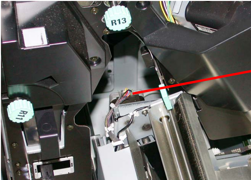
Figura 1. Posición del motor del recorrido del papel del folleto
