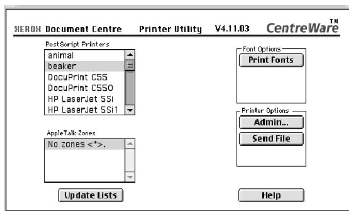
Figur 5-1: Macintosh skrivarverktyg
