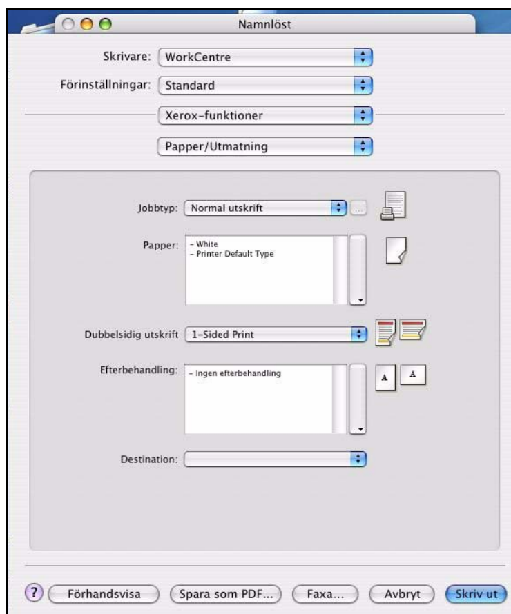
Figur 3-1: Dialogrutan Skrivardrivrutin
