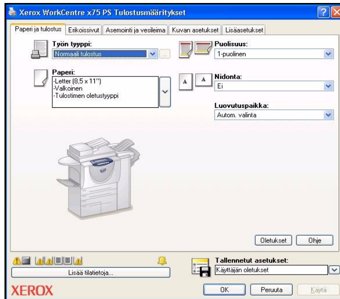
Kuva 3-1: Ajurin käyttöliittymä
