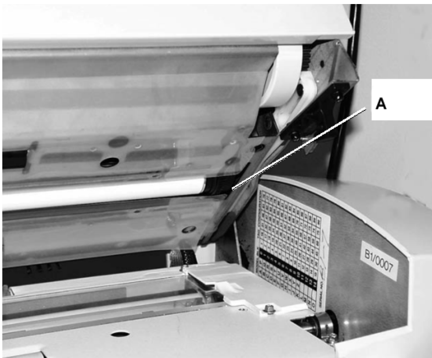
A: Calibration Roll Drive Gear
