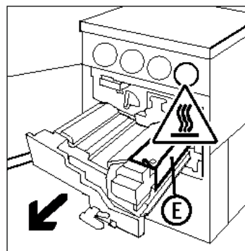
Figuur 42: De papierbaanmodule naar buiten trekken
