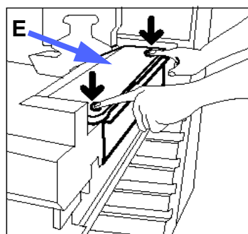
Figuur 44: Het reinigingsweb ontgrendelen
